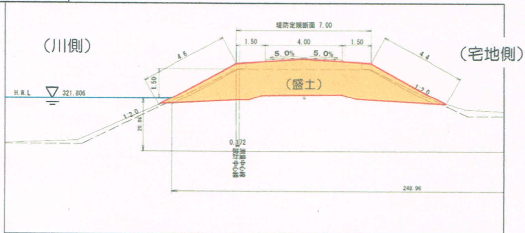
(横断図)
